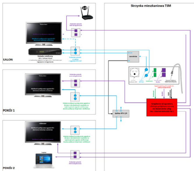
Rys. 1. Instalacja teletechniczna w mieszkaniach na osiedlu przy ul. Sklepowej 22
